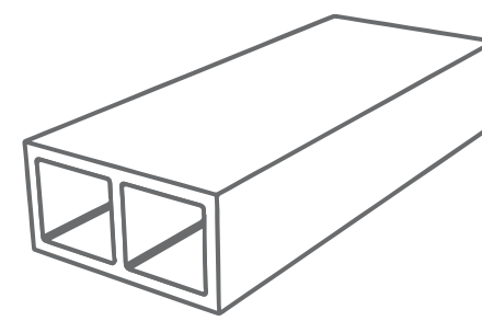
Perfil Annapurna 80 80x40x3000 mm
