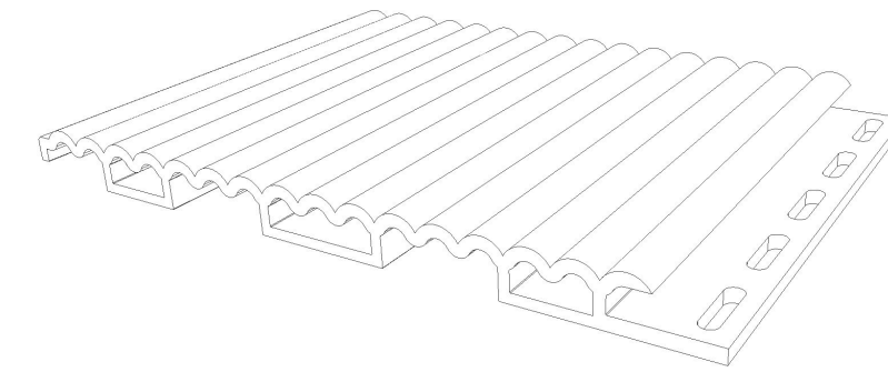
Perfil Aris Onna 217,5 x 15 x 3000 mm
