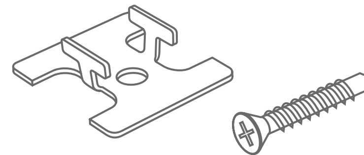
Clip de fijación / Tornillo acero inox. 40 x 45 mm / 4,2 x 25mm
