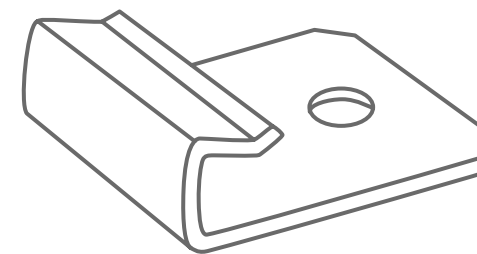
Clip de inicio inox 32 x 29 x 10mm
