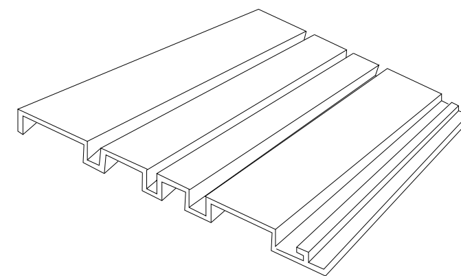
Perfil Aris Horizon 269,5x15x3000 mm
